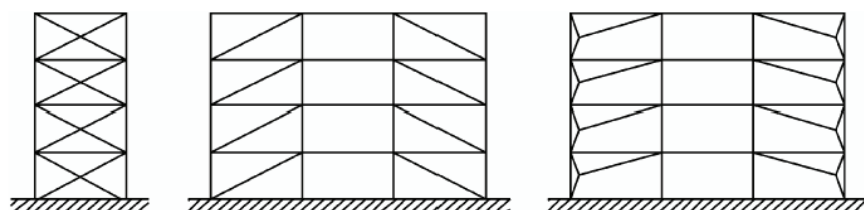
Controventi concentrici a diagonale tesa attiva
